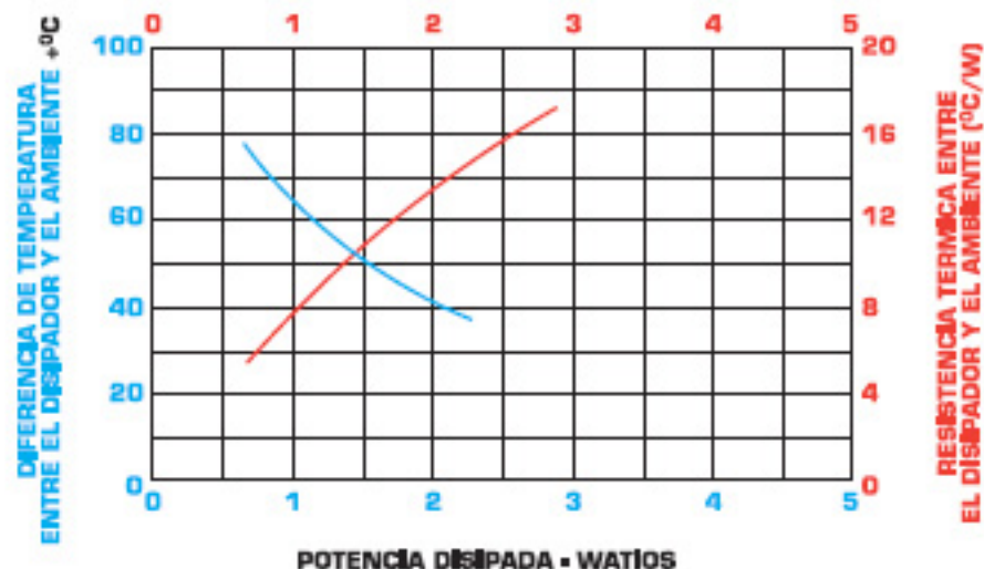
CARACTERÍSTICAS CON CONVENCIÓN NATURAL Y FORZADA VELOCIDAD DEL AIRE • METRO/SEGUNDO
