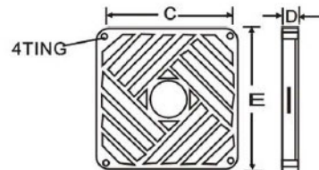
Fan Guard
