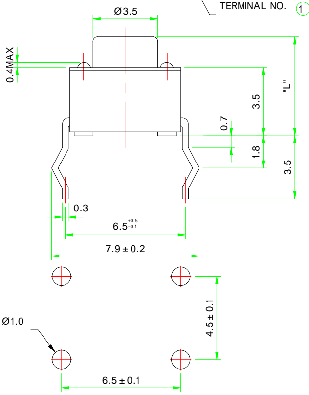
P.C.B DIMENSION
