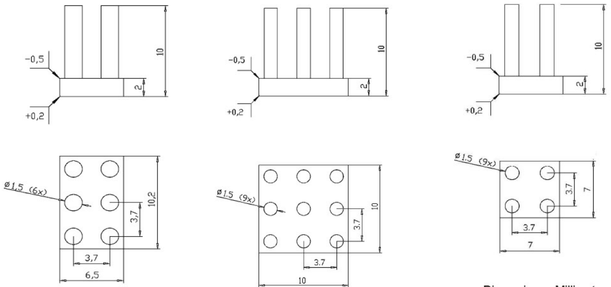
Dimensions : Millimetres
