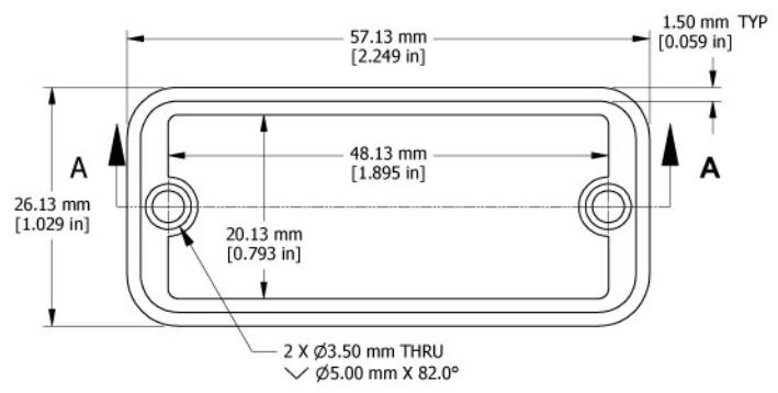
OPEN BEZEL
